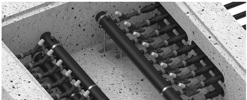
Beispielbild Erdsondenverteilerschacht in Bodenplatte für ein MFH
